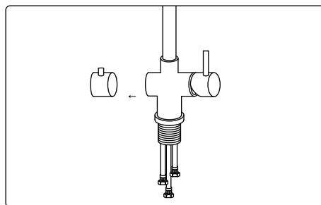
2. Verwijder de hendel
